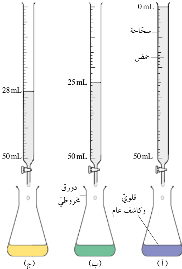
استخدام سّحّاحة لإضافة حمض إلى دورق مخروطيّ يحتوي على قلويّ.
