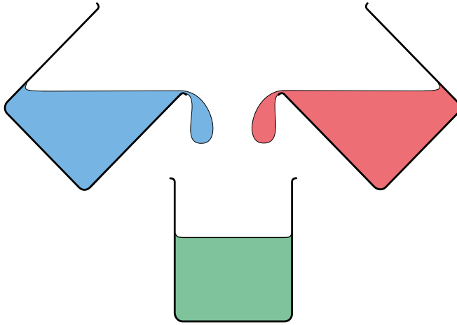
خلط حمض مع قلويّ لتحضير محلول متعادل
