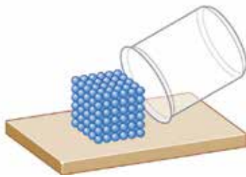
المواد الصلبة لا يمكن أن تتدفق.
