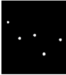
نجوم كوكبة كاسيوبيا Cassiopeia
