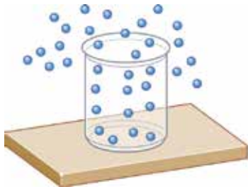
المواد الغازية تتدفق وتنتشر.
