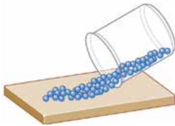
المواد السائلة تتدفق.
