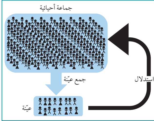
الشكل ٥-٢ رسم تخطيطي يمثل جماعة أحيائية وعينة ممثلة لها.
