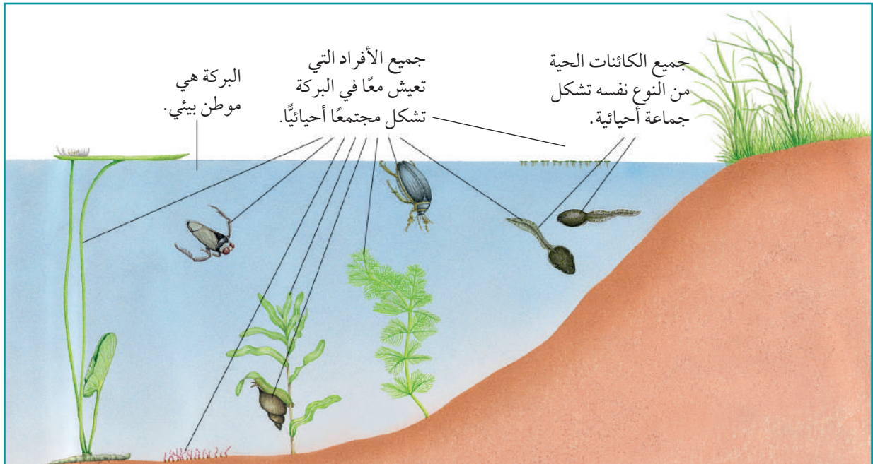
الشكل ١-٤ البركة والكائنات الحية التي تعيش فيها تشكل نظاماً بيئياً.
