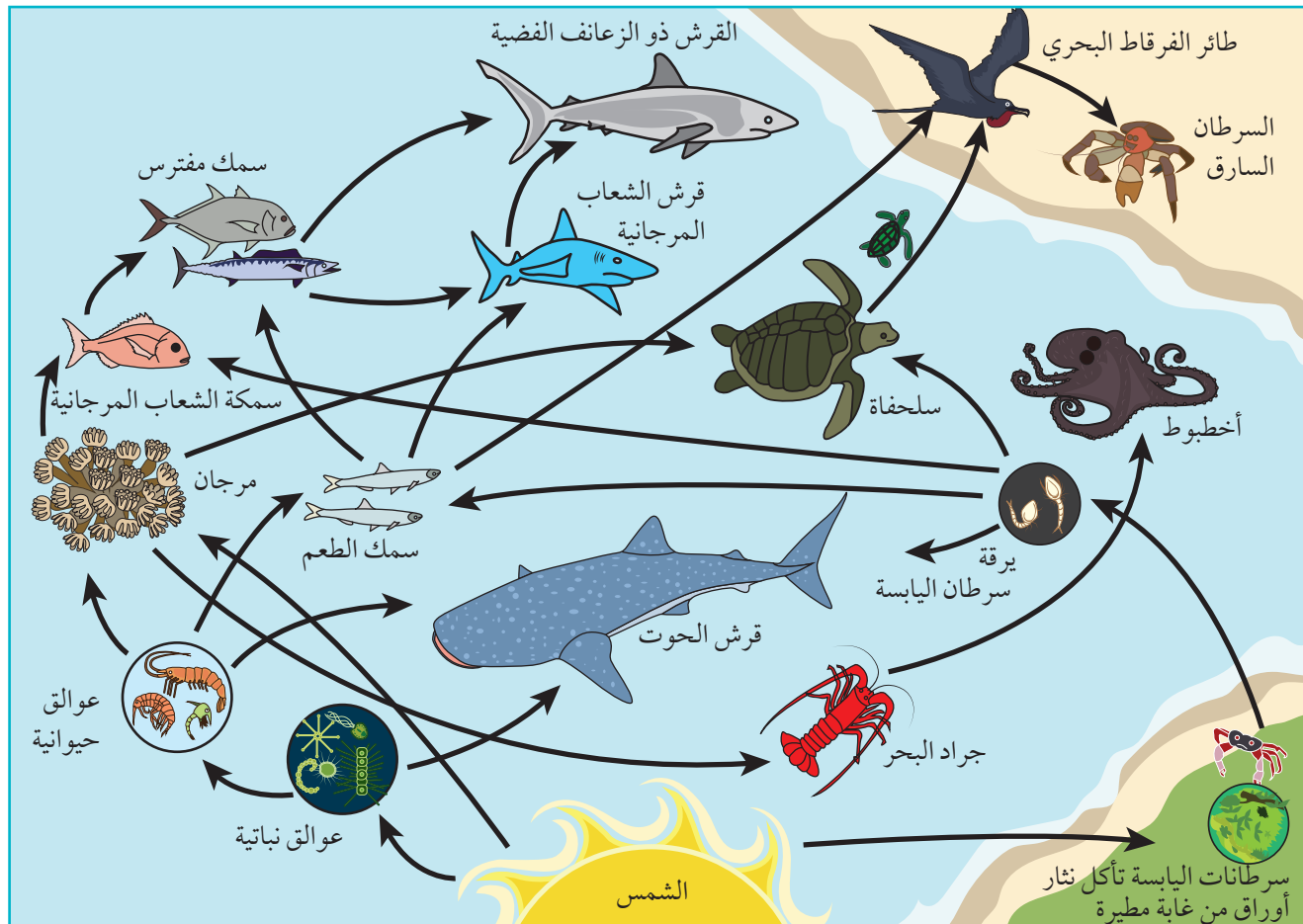
الشكل ٨-١ مثال على الشبكة الغذائية التي توضح التعقيد في مسارات الطاقة مع مصادر غذاء مختلفة لكائنات حية متنوعة.
