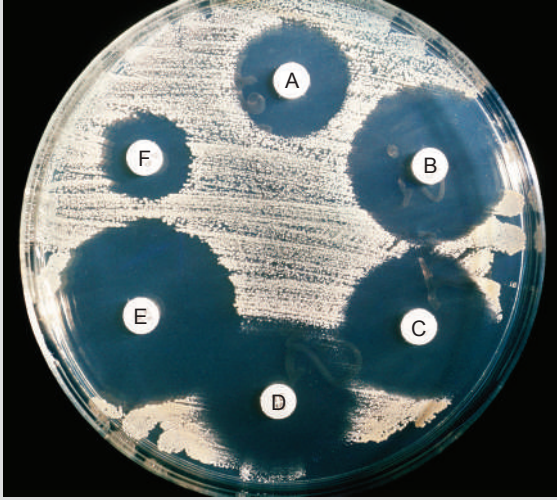
الصورة ١٦-٢ تأثير المضادات الحيوية التي تنتجها ستة أنواع جديدة من الإسفنج البحري (A-F).
