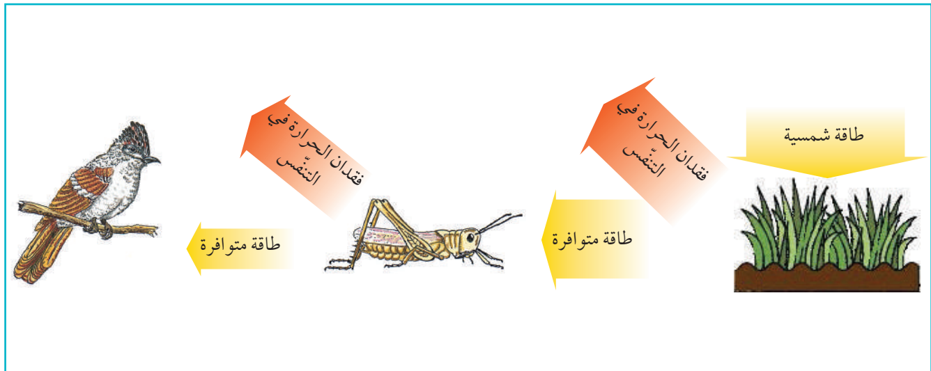
الشكل ١-٧ يوضح سلسلة غذائية تدفق فيها الطاقة من المنتجات (النباتات) إلى المستهلك الأولي (الجندب)، ثم إلى المستهلك الثانوي (صائد الذباب).
