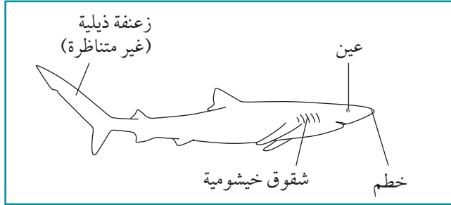
الشكل ٤-٢ رسم بيولوجي لقرش أزرق.
