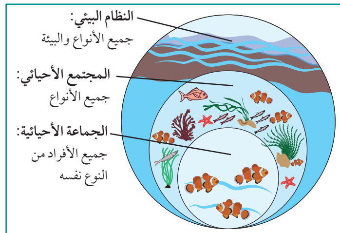
الشكل ١-٥ العلاقات بين الجماعات الأحيائية والمجتمعات الأحيائية والنظم البيئية.
