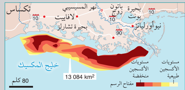
الشكل ٣-١٣ متوسط المساحة لمنطقة ميتة في سنة 2018 م.
