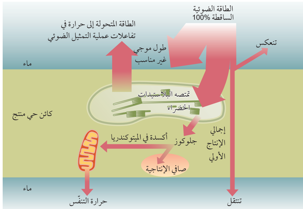
الشكل ٢-٣ مصير الطاقة الضوئية الساقطة على المنتجات في المحيط.
