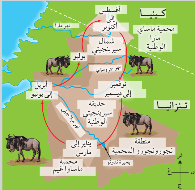
الشكل ١-١٤ طرق هجرة القطعان الكبيرة.
