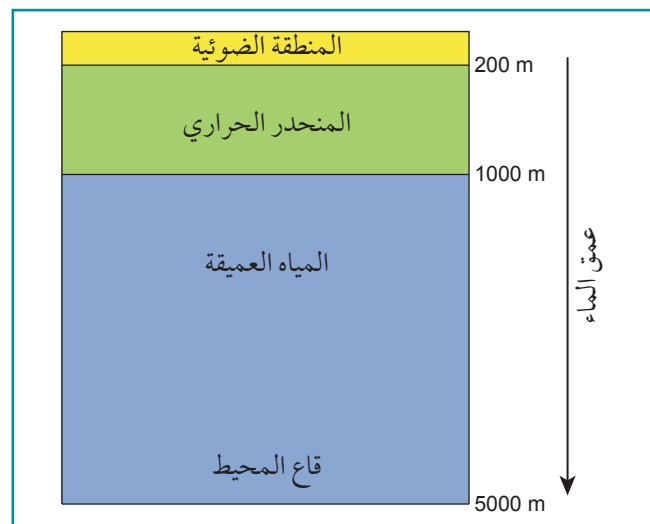
الشكل ٣-١ طبقات الماء في المحيط.
