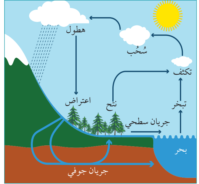
الشكل ١-١ دورة الماء.
