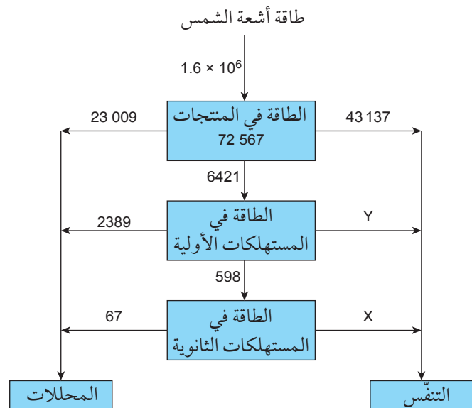
الشكل ٧-٣ مثال عملي على الرسم التخطيطي لتدفق الطاقة (الوحدات المستخدمة بـ kJ/ m 2 year).
