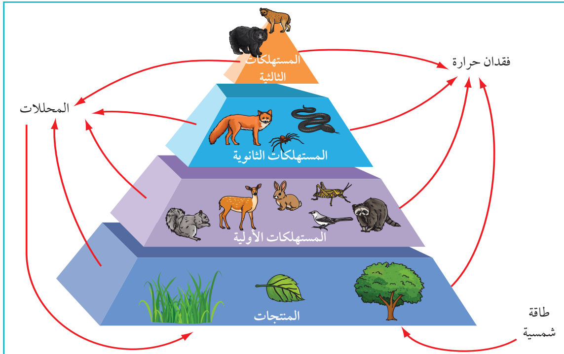
الشكل ١-٦ هرم بيئي يوضح كيف يتوافق الصعود عبر المستويات الغذائية مع انخفاض مقدار المغذيات المتوفرة. يتم تمرير 10% فقط من الطاقة إلى المستوى التالي، ما يقلل من كمية الطاقة المتوفرة أثناء صعود الهرم.
