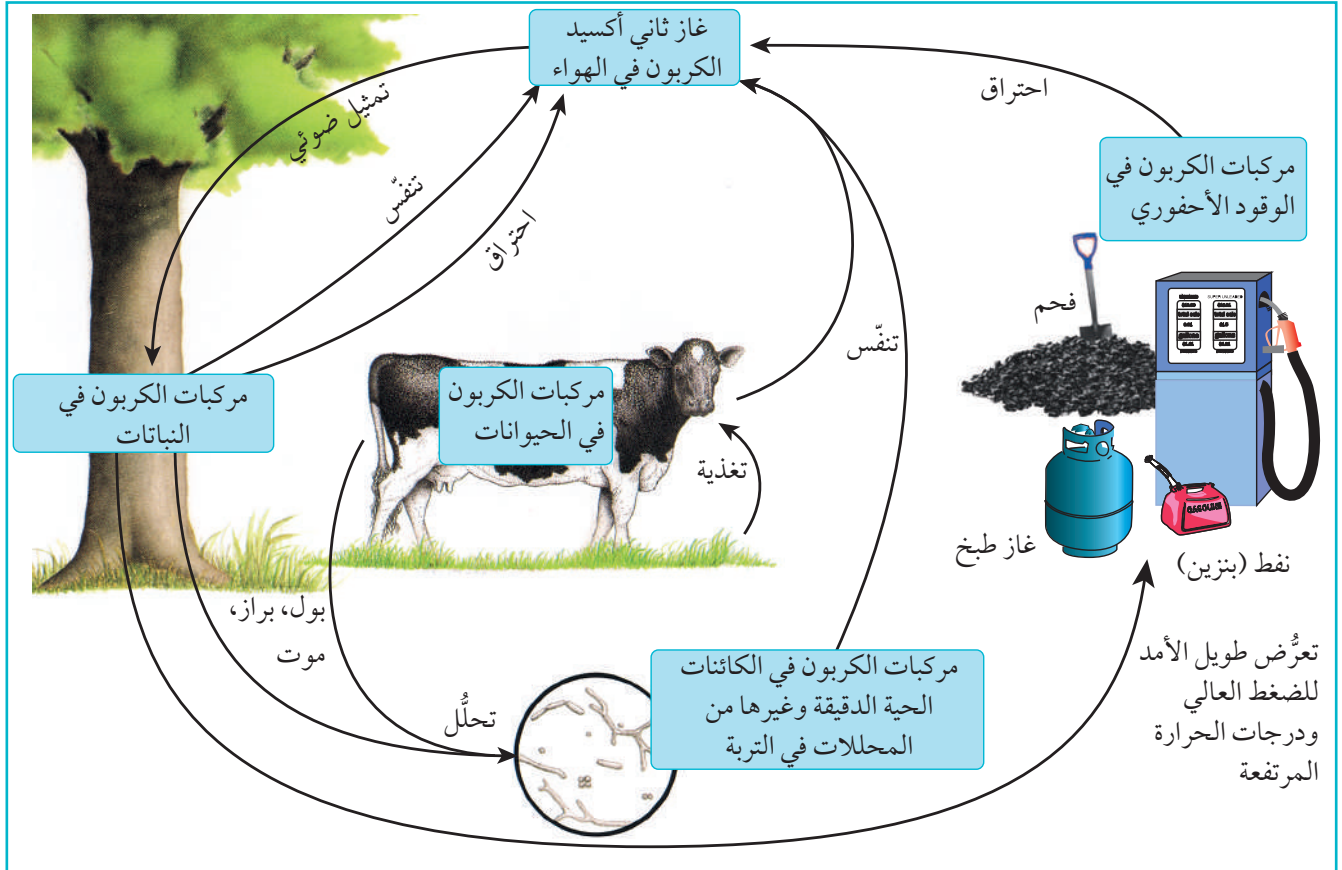
الشكل ٩-١ دورة الكربون، توضح كيف يمكن أن ينتقل ثاني أكسيد الكربون من مخزن إلى آخر في فترة زمنية قصيرة نسبيًا (أسابيع، أيام، وحتى ساعات).
