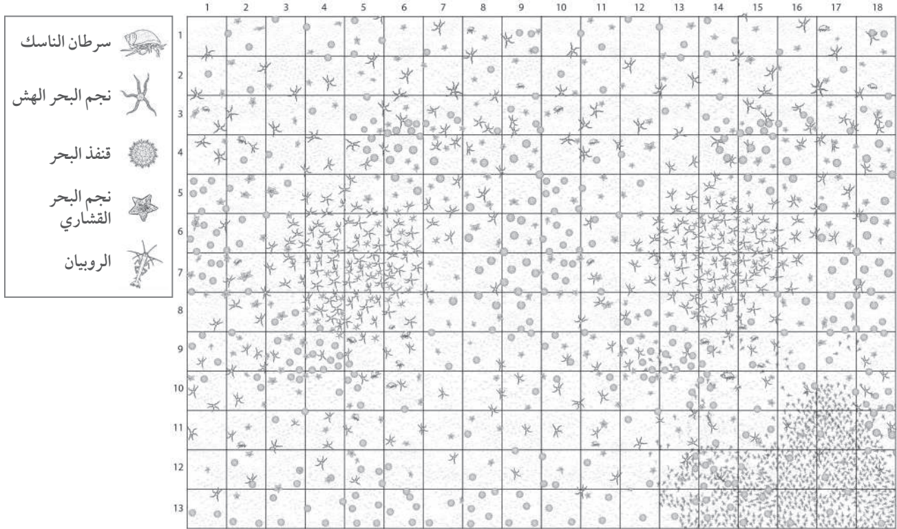
الشكل ١١-٢ الموطن البيئي لقاع البحر.
