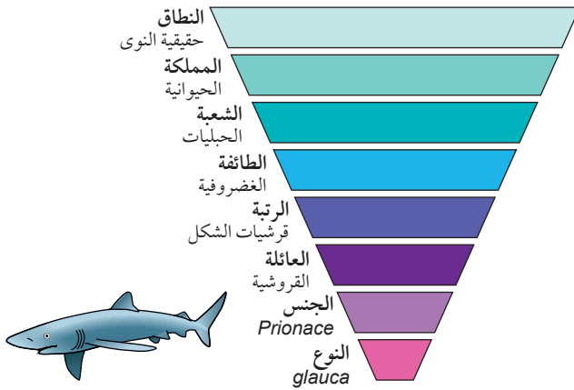
الشكل ٤-١ التسلسل الهرمي التصنيفي للقرش الأزرق Prionace glauca .
