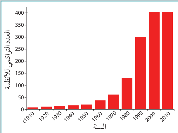
الشكل ١٢-٣ أعداد المناطق الميتة على امتداد العقود.
