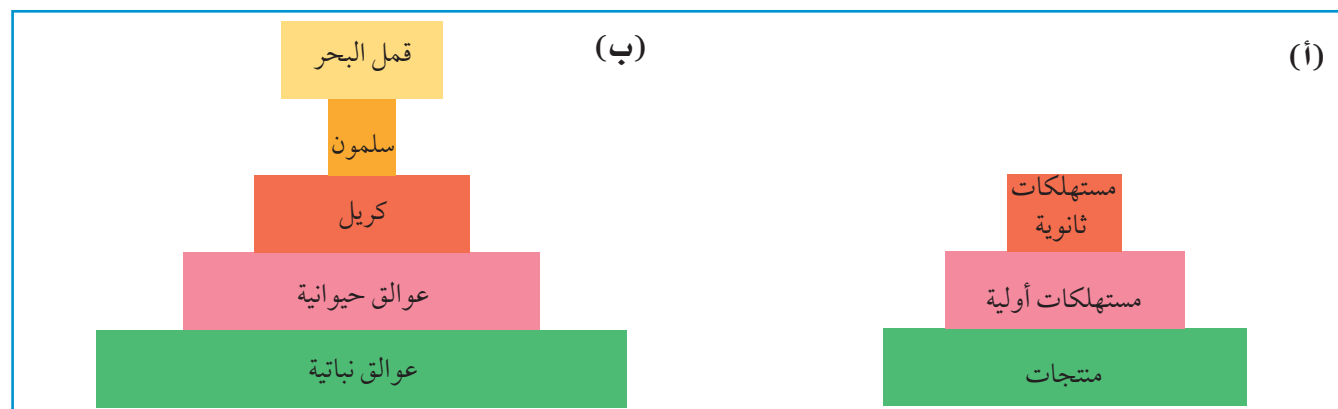
الشكل ٣-٤ (أ) هرم أعداد عام، (ب) هرم الأعداد للنظام البيئي البحري يبين طفيليات صغيرة تتغذى على سمكة كبيرة.
