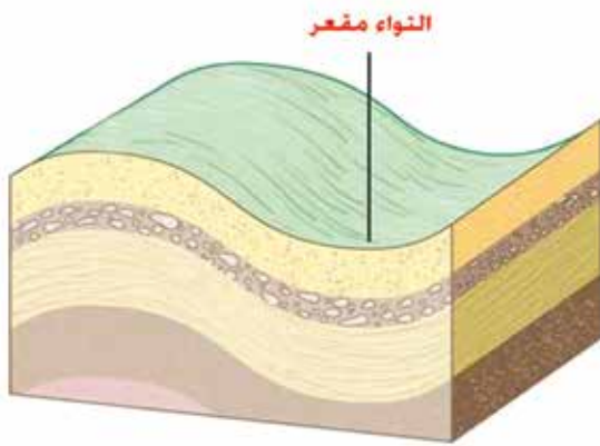
الشكل (١٧): التواء مقعر
