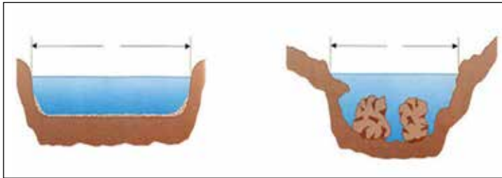
الشكل (٢٤) : النحت الرأسى والأفقي لمجرى النهر
