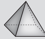
هرم مربع القاعدة
