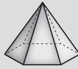
هرم سداسي القاعدة
