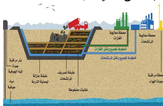
الشكل (٨) رسم توضيحي لمردم هندسي
