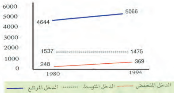
الشكل (٤): متوسط نصيب الفرد من الطاقة في العالم.
