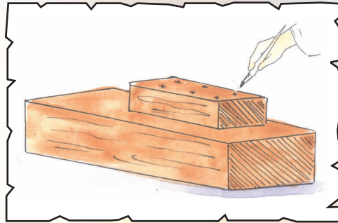
الشكل ( ٤ ) : تحديد أماكن وضع المسامير أو البراغي .
