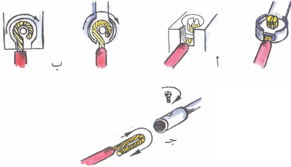
الشكل (٢٢) : طرق تثبيت السلك بمسمار القابس .
