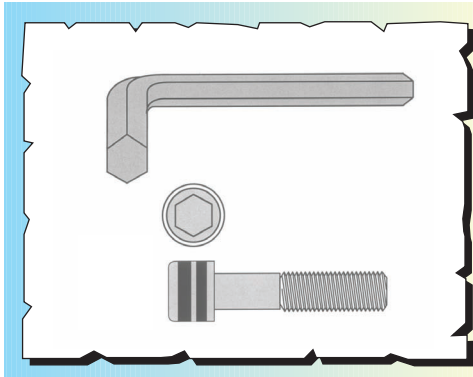
الشكل (٢) : برغي يستخدم في تثبيت قطع الأثاث الخشبي الجاهز مع أداة تثبيته .
