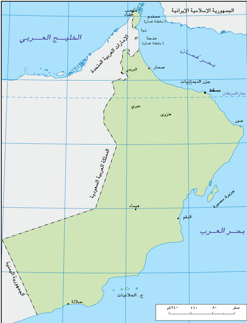
شكل (٢٧) خريطة سلطنة عُمان
