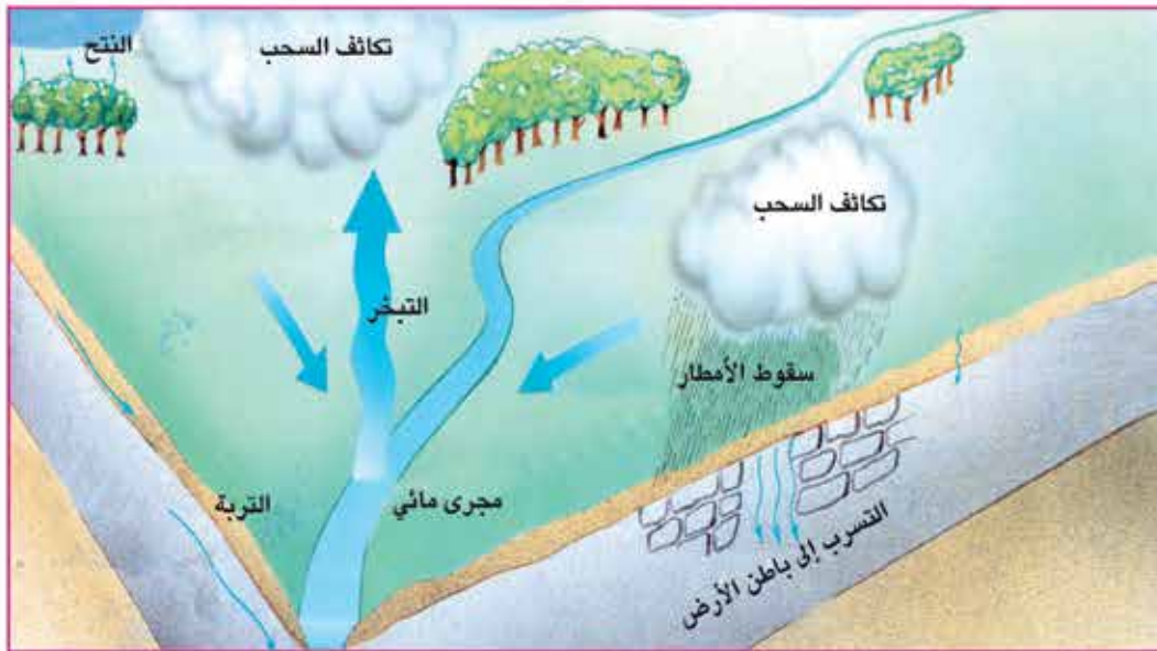
شكل (٢) الدورة المائية
