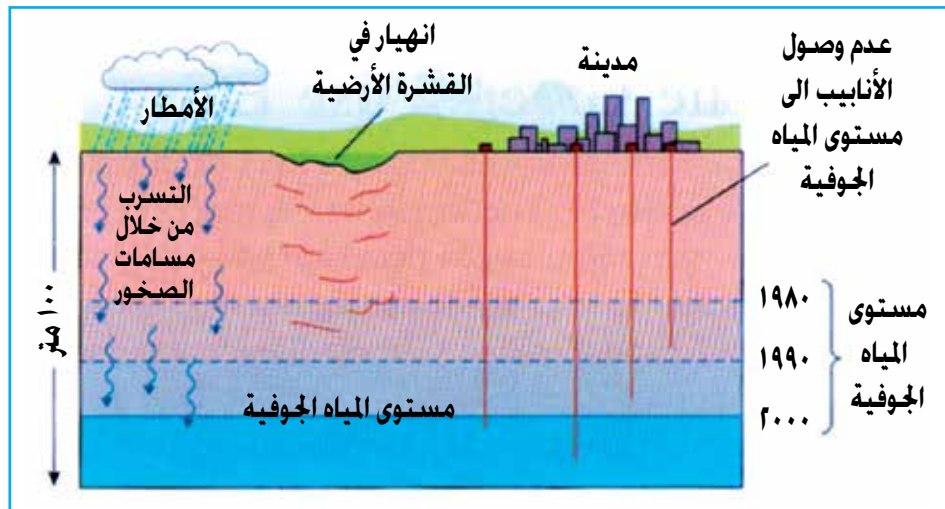
شكل (٢١) انخفاض منسوب المياه الجوفية
