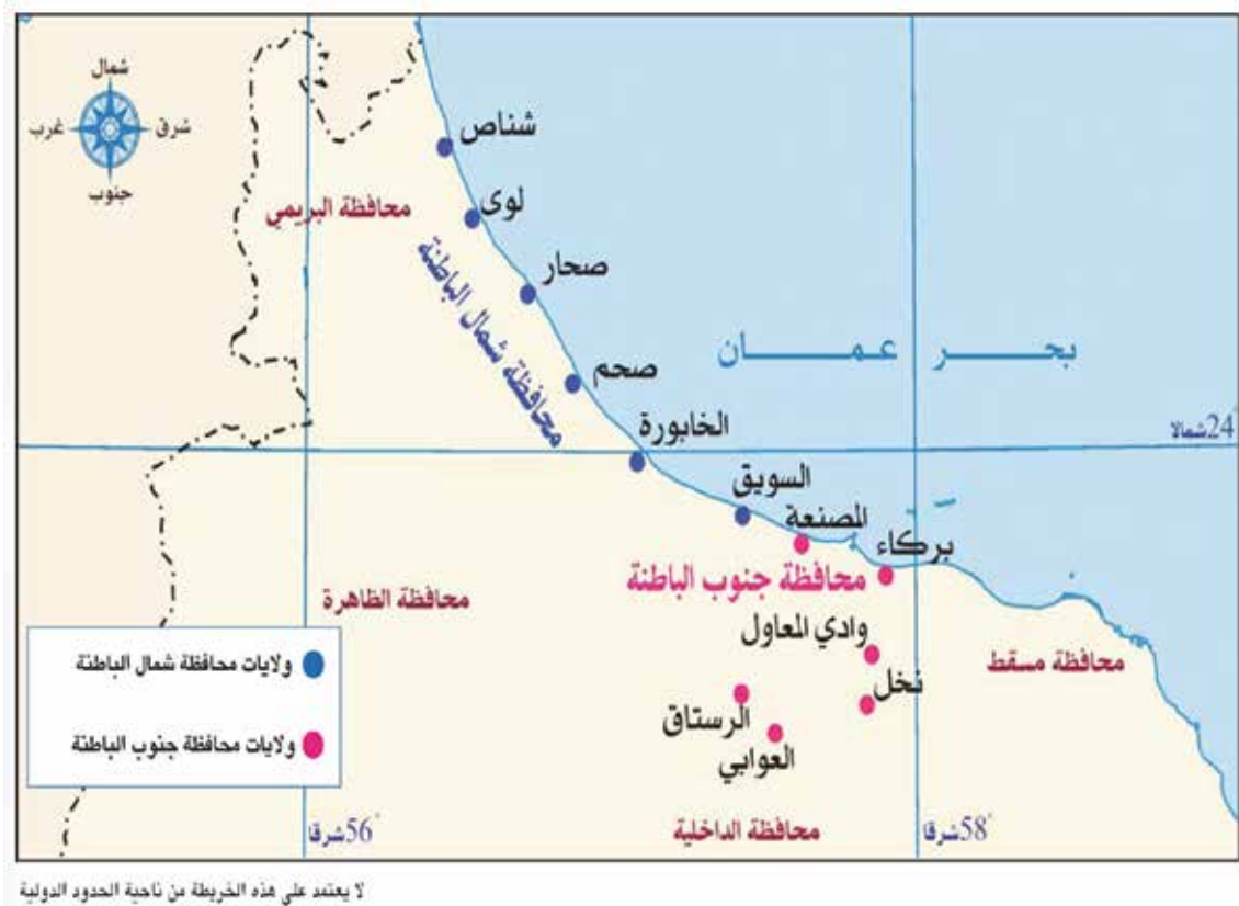
شكل (٢٥) خريطة ساحل الباطنة بسلطنة عُمان
