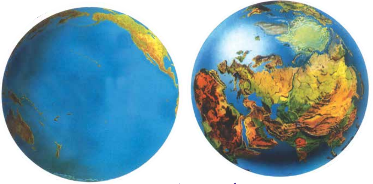
شكل (١) توزيع اليابس والماء
