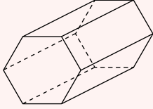
المنشور السداسي
