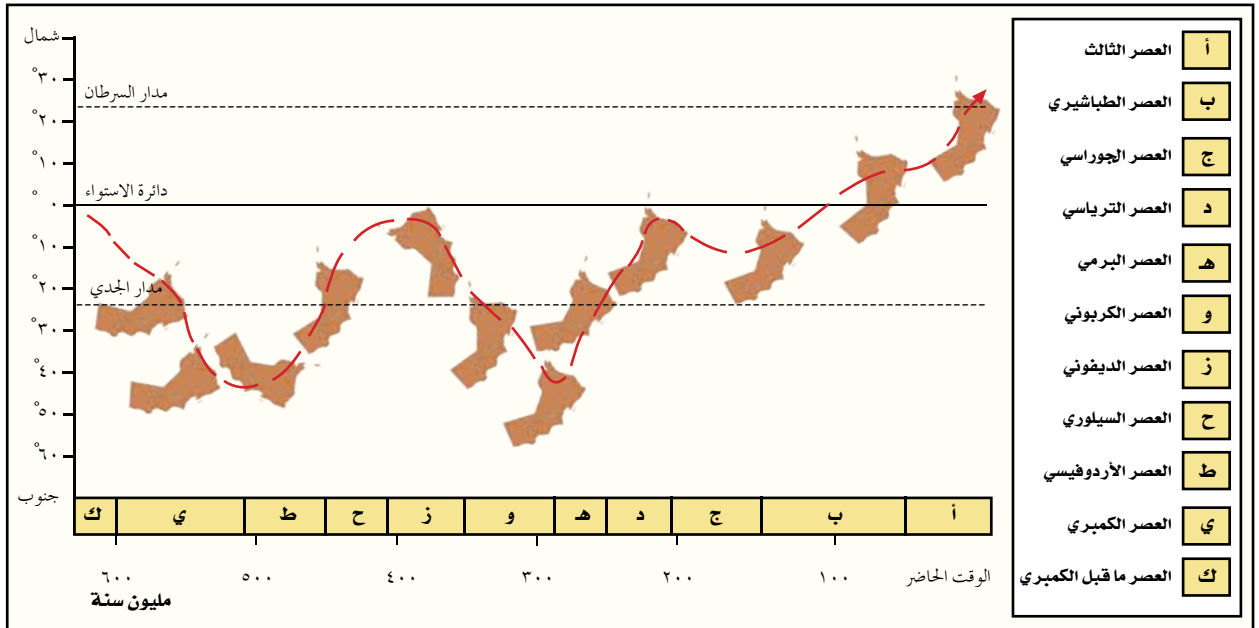
الشكل (٤) مسار عُمان خلال العصور الجيولوجية المختلفة
